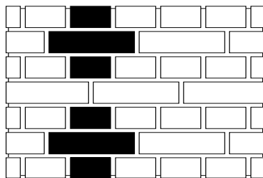
▲ Kreuzverband
