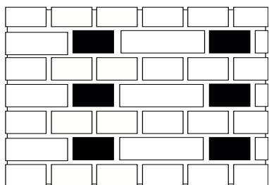
▲ Holländischer Verband
