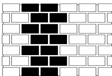
▲ Kopfverband/Binderverband
